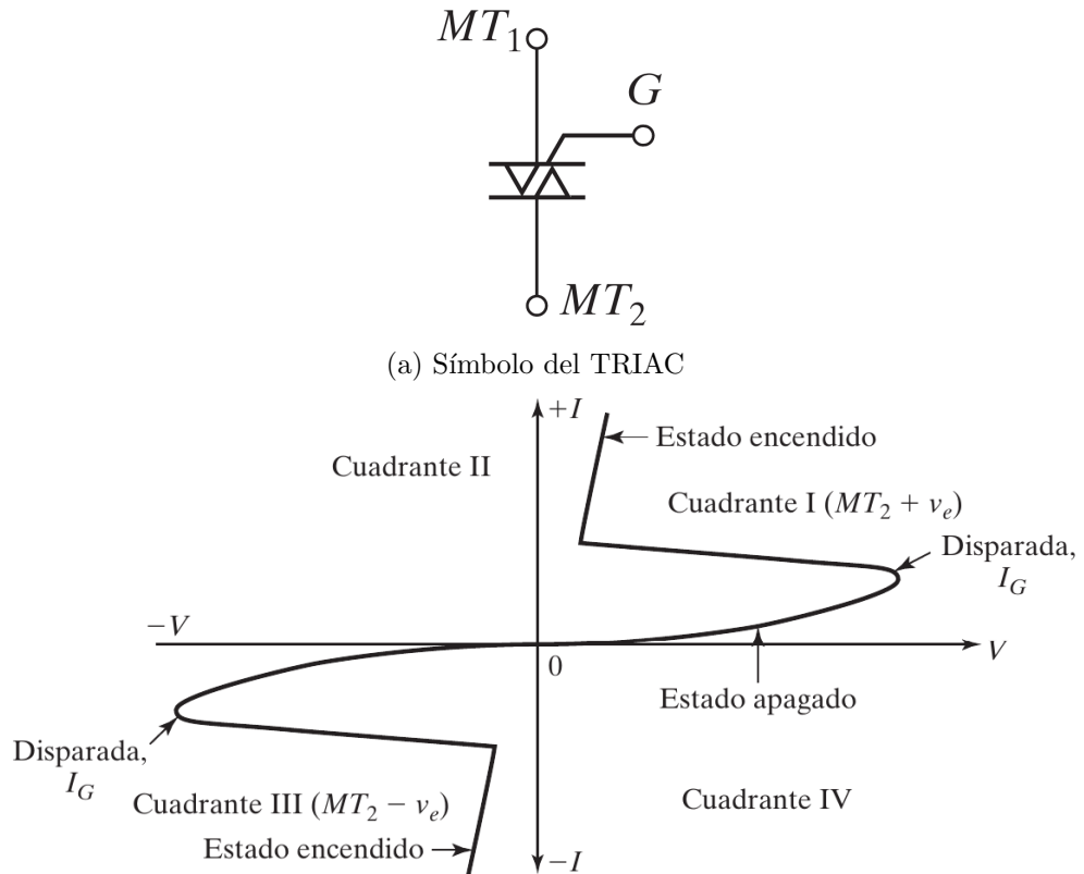
(b) Curva corriente-voltaje de un TRIAC
